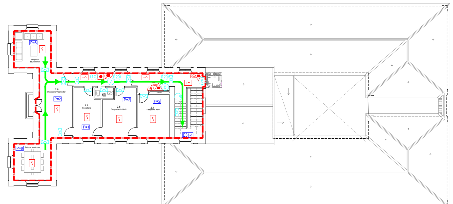
PLANTA PRIMERA
